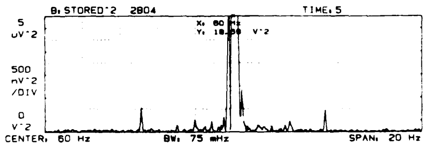
(d) slip=0.04
