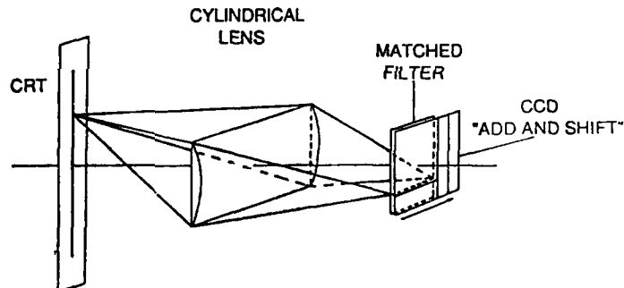
Fig.1. OPTICAL PROCESSOR.
