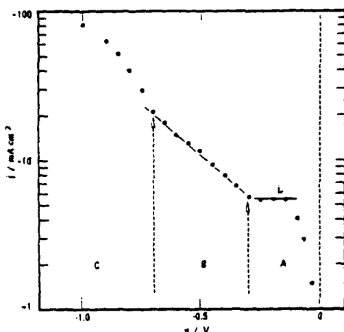
Fig. 1 Tafel plot
