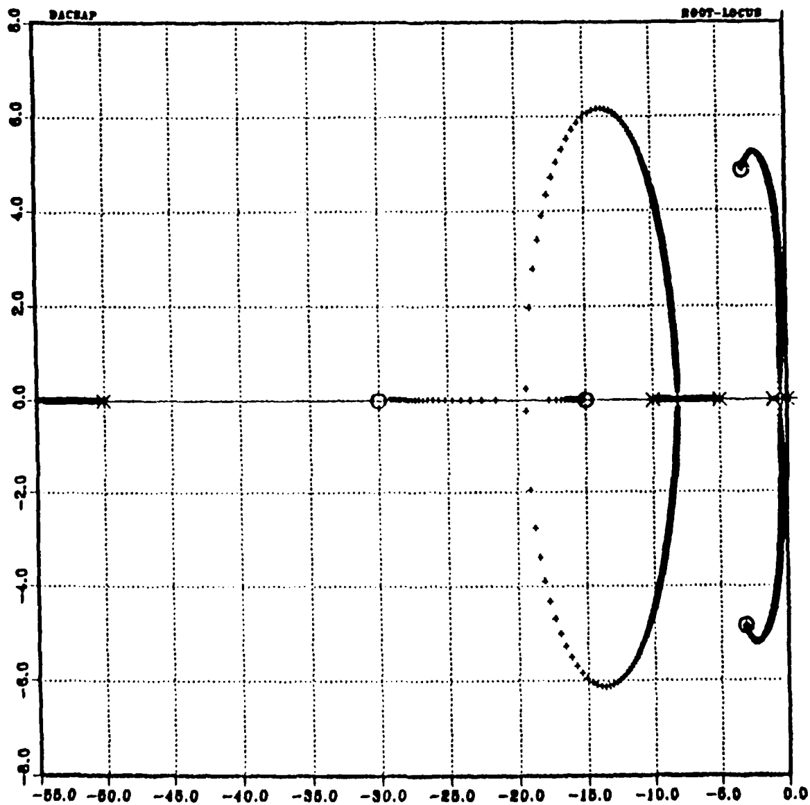
Figure 58. Offsetting The Zeros. Desired Roots; -3.000 \pm j5.000 , -15.000 , -30.000
