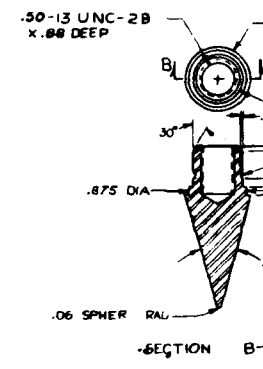
⑤ CONE
