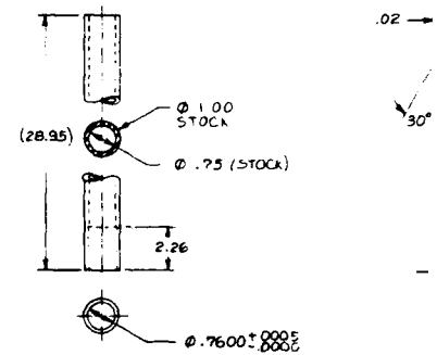
⑨ GUIDE TUBE
