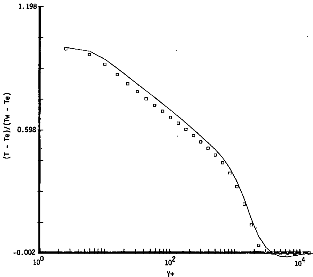
f. Temperature profile (wall scaling)
