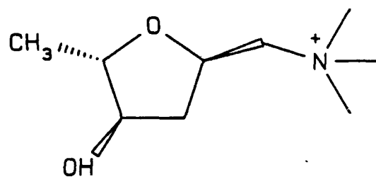
d. allomoscarine
