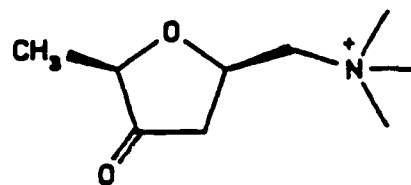
cis-Muscarone
