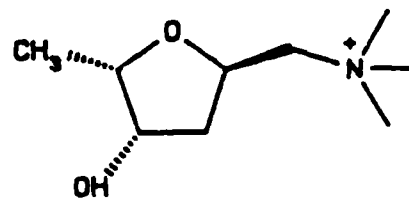
Epiallomuscarine
