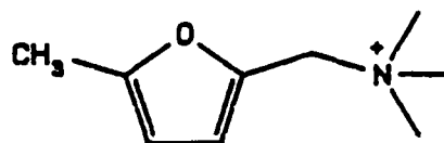
5-Methylfurfurmethide
