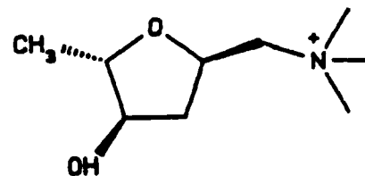
Allomuscarine
