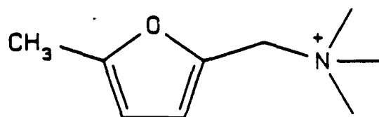
h. 5-methylfurfmethide
