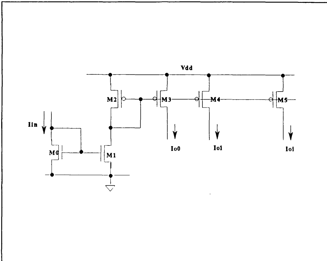
Fig. 3.1 Input replicator
