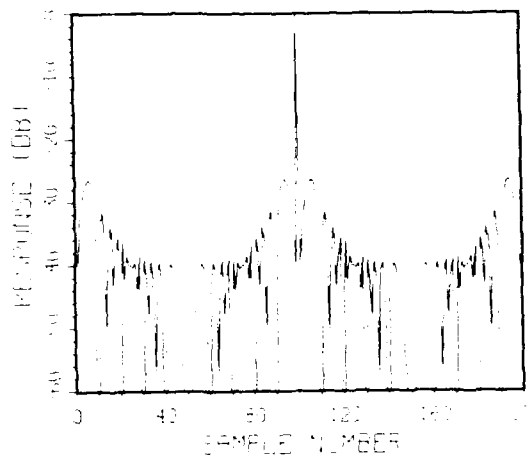
Fig. 3 — 100 element P4 code ACF
