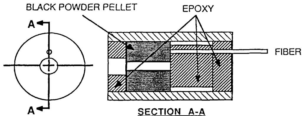
Figure 3. Test primer
