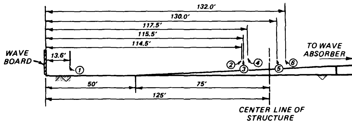
a. Profile
