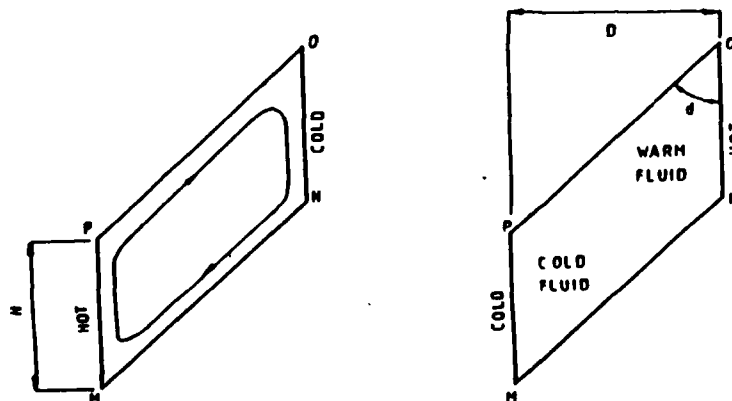
Figure 1. Thermal rectifier
