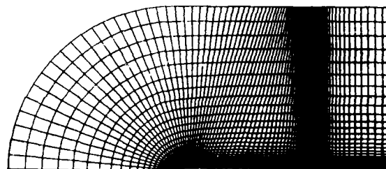
a. Supersonic Grid
