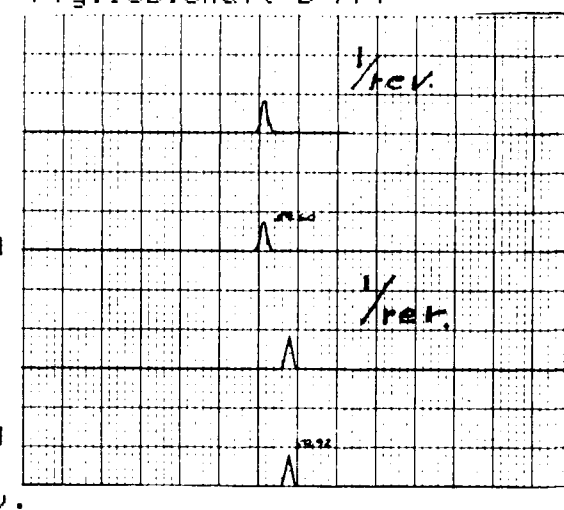
60 +/- 2.HZ Fig.19b:Shaft-B FFT Zoom
