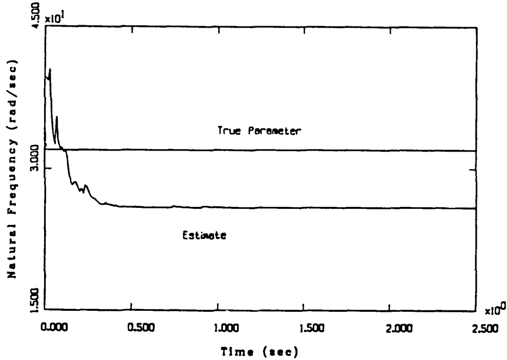
Figure 22. Parameter Estimation Convergence
