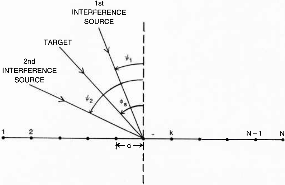
Fig. 1 — Array geometry
