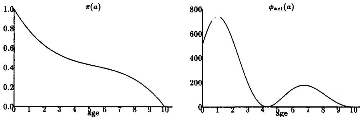
Fig 2. Life Table and Actual Initial Distribution
