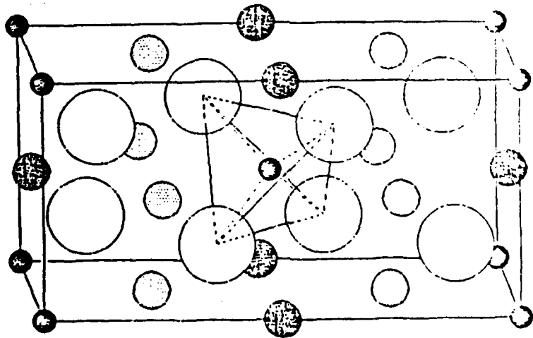
(a) Stannite
