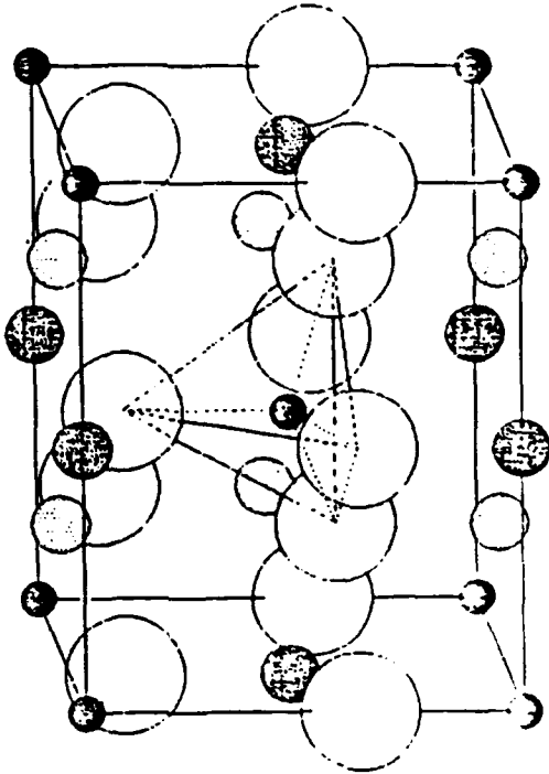
(b) Wurtz-Stannite
