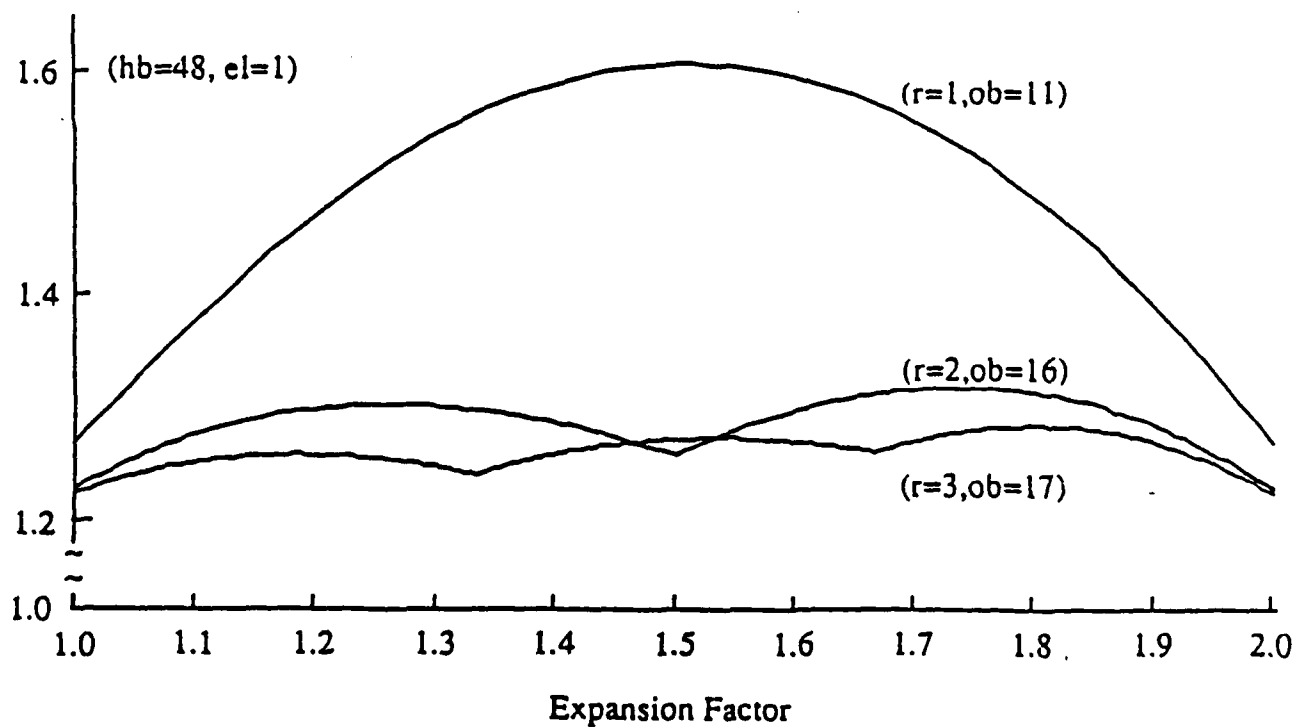
Figure 5.2 DRSAM successful search cost ( auf = 0.91 )
