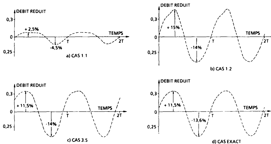
Fig. 6 - Débit à l'entrée d'un canal de la roue mobile.
