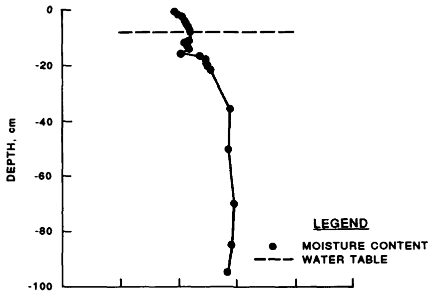
a. Moisture profile, Site 1, 13 August 1987
