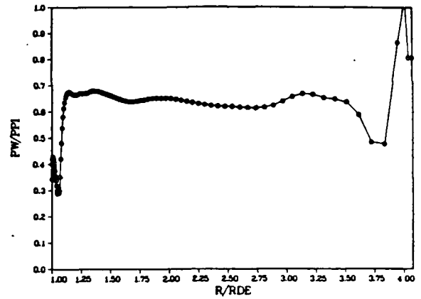
N=40K PW/PPI CSB ACTUAL INFLOW 47%NSR
