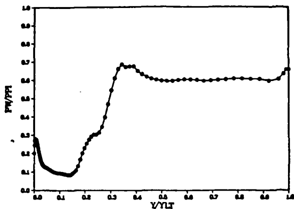
N=150K PW/PPI ACTUAL INFLOW 60%NSR
