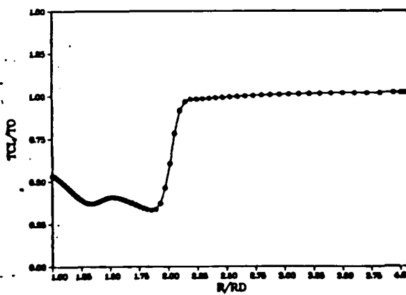
N=225K TCL/TO ACTUAL INFLOW 47%NSR
