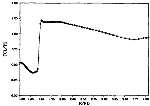
N=40K TCL/TO CSB ACTUAL INFLOW 47%NSR
