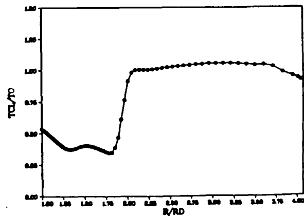
N=50K TCL/TO ACTUAL INFLOW 47%NSR
