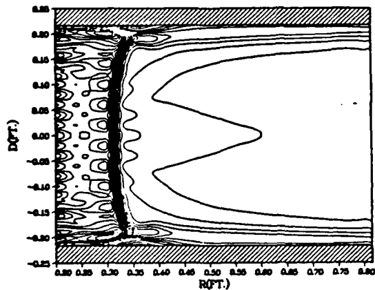
N=185K ACTUAL INFLOW 60%NSR WBB=.195
