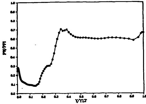
N=300K PW/PPI ACTUAL INFLOW 60%NSR
