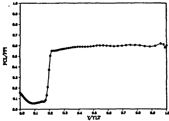
N=300K PCL/PPI ACTUAL INFLOW 60%NSR
