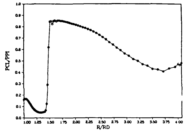
N=40K PCL/PPI CSB ACTUAL INFLOW 47%NSR
