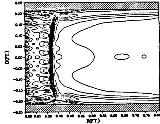
N=115K ACTUAL INFLOW 60%NSR WBB=.195
