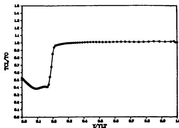
N=350K TCL/TO ACTUAL INFLOW 60%NSR
