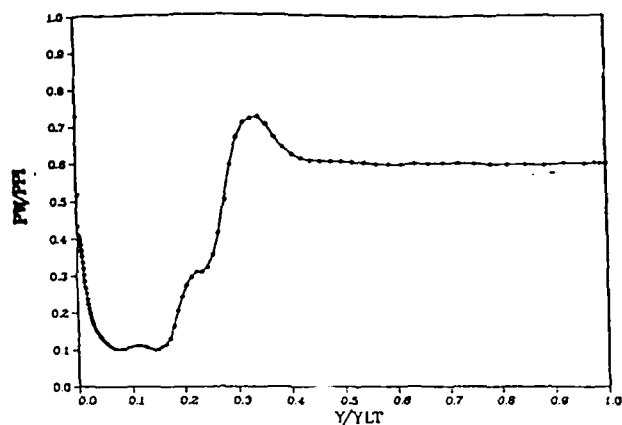
N=475K PW/PPI ACTUAL INFLOW 60%NSR
