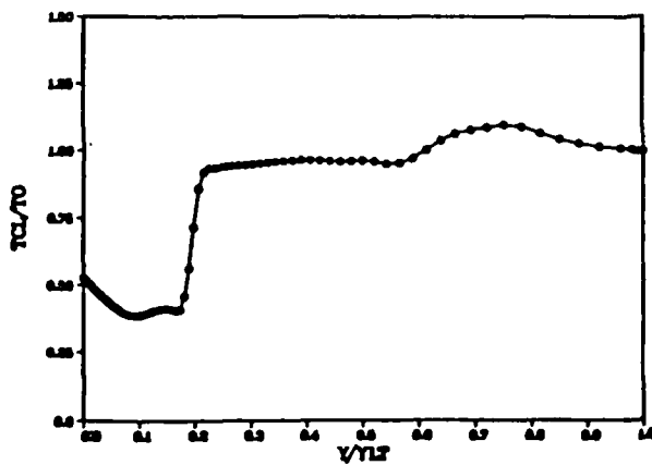
N=100K TCL/TO ACTUAL INFLOW 60%NSR
