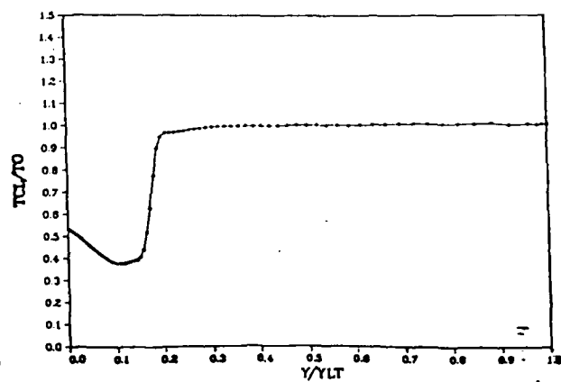
N=475K TCL/TO ACTUAL INFLOW 60%NSR
