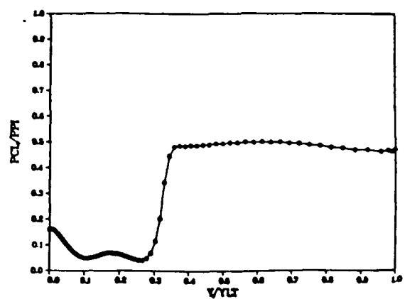
N=350K PCL/PPI XK2 47%NSR
