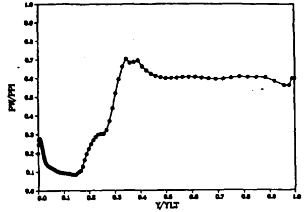
N=325K PW/PPI ACTUAL INFLOW 60%NSR
