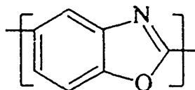
Poly(2,5(6)-benzoxazole)--ABPBO
