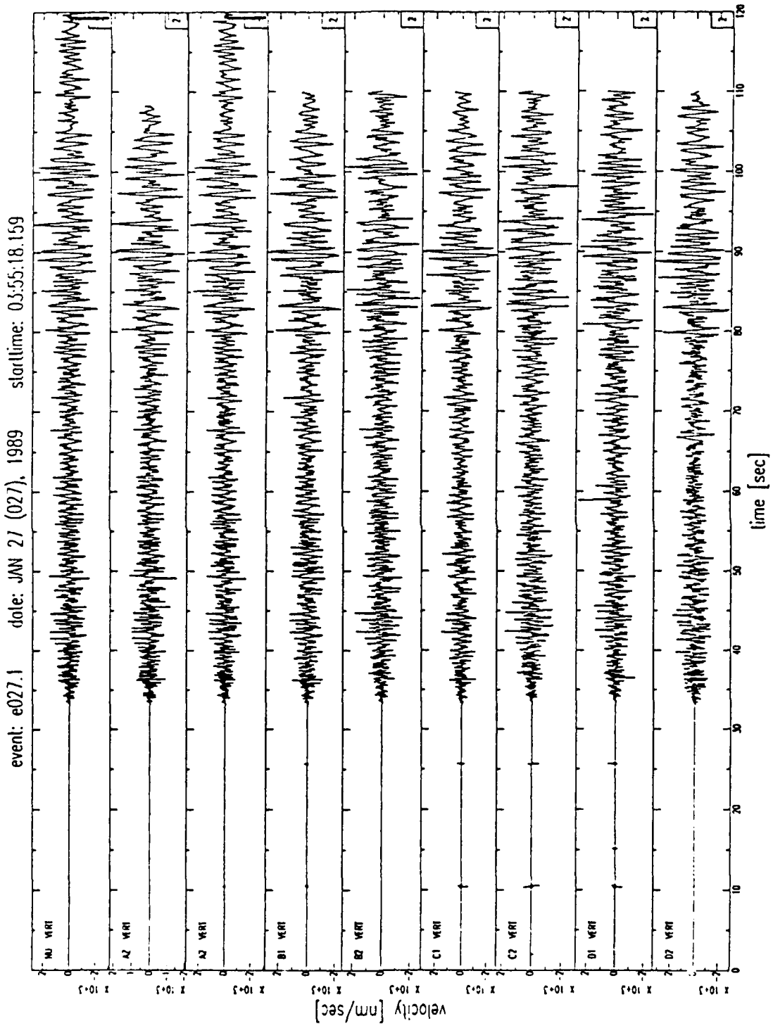
Fig. 23 : event 3 : Hungary 01/27/1989 03:55:05.6
