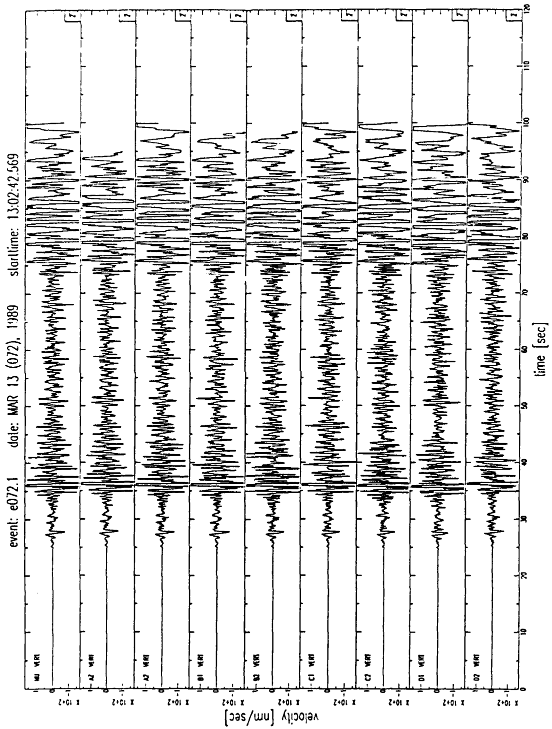
Fig. 29 : Event 9 : GDR 03/13/1989 13:02:18.2
