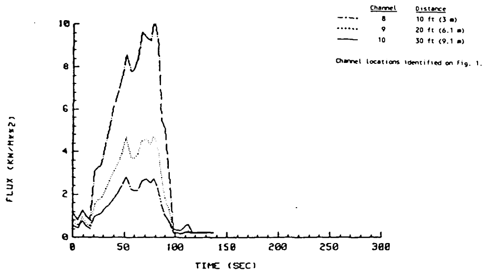
SFS 019 RADIOMETER PLOTS
