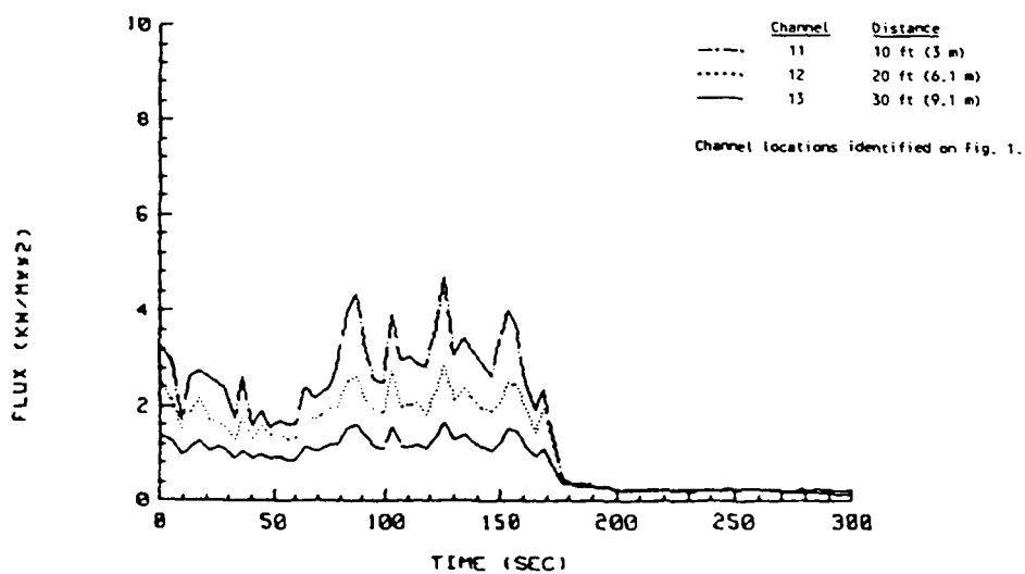
SFS 006 RADIOMETER PLOTS
