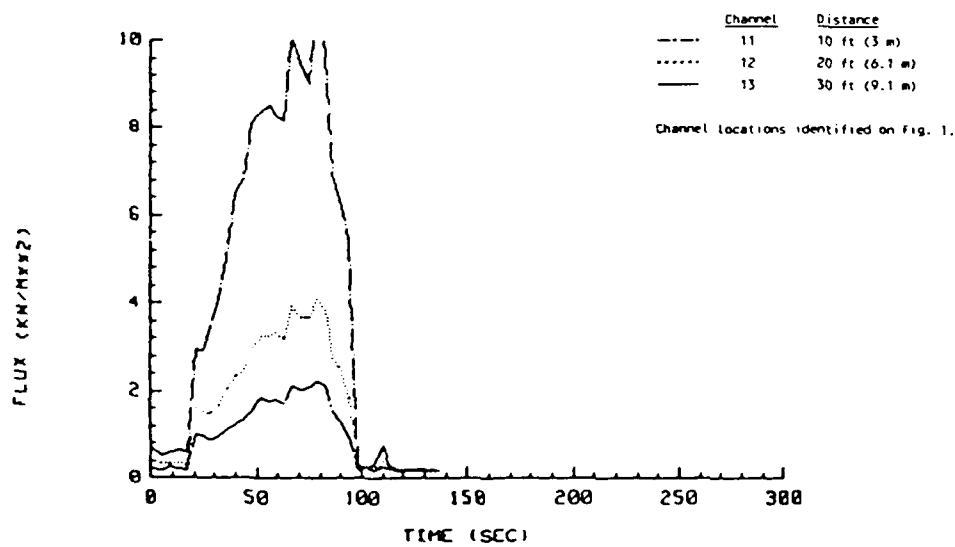
SFS 019 RADIOMETER PLOTS
