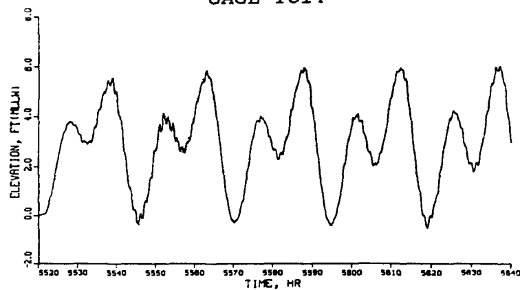
GAGE TC17
