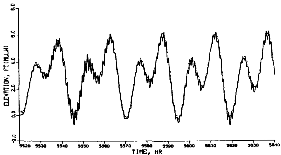
TIDE GAGE TG 3
