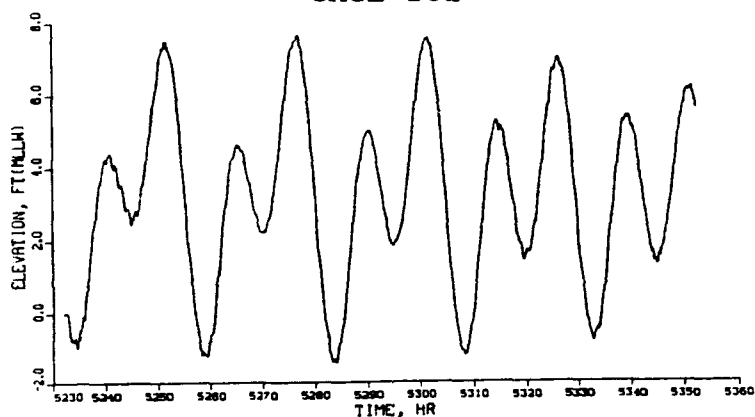
GAGE TC3
