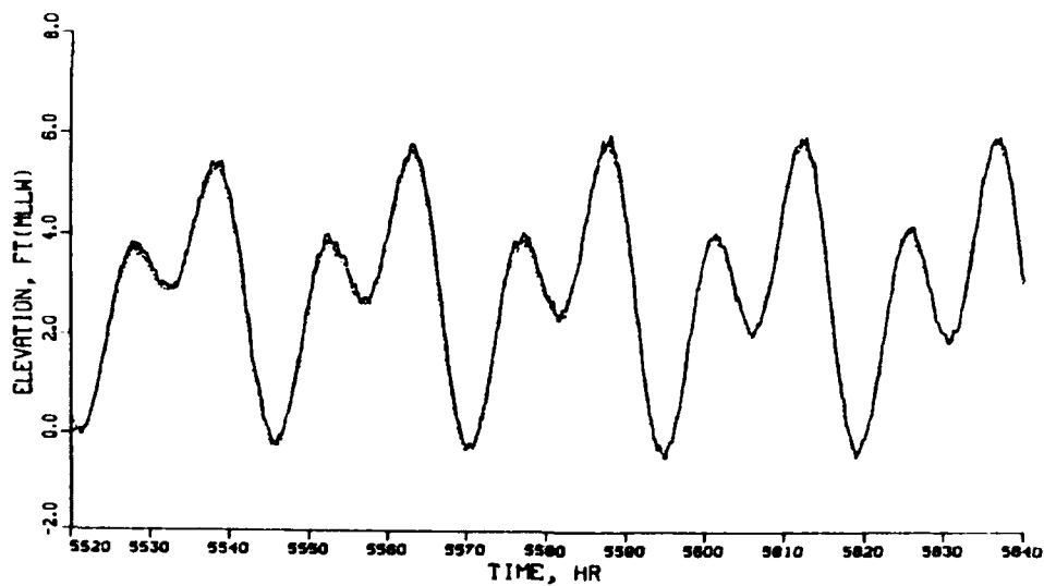
TIDE GAGE TG 7
