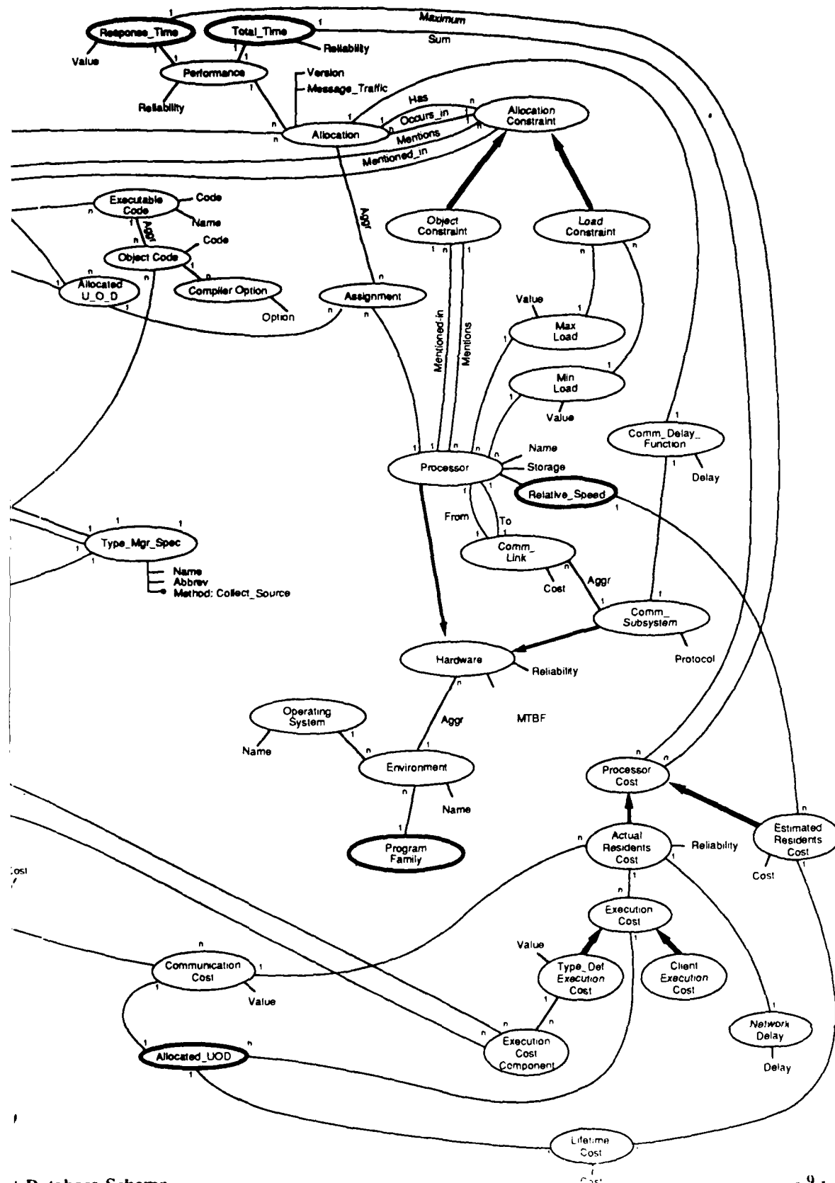
Database Schema
