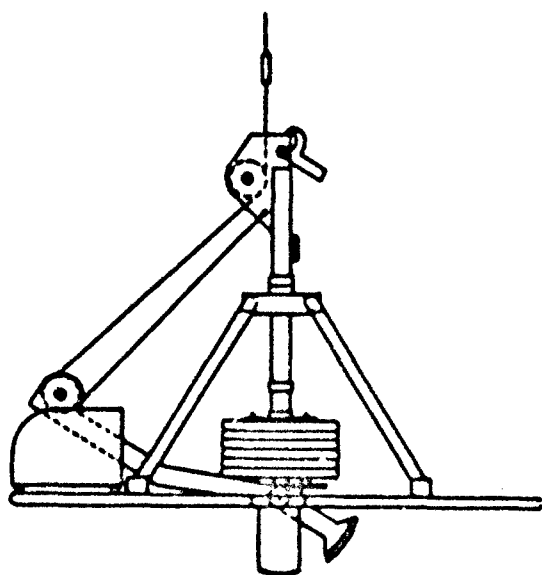
a. Reineck box sampler
