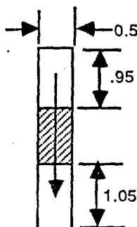
SEC A-A
