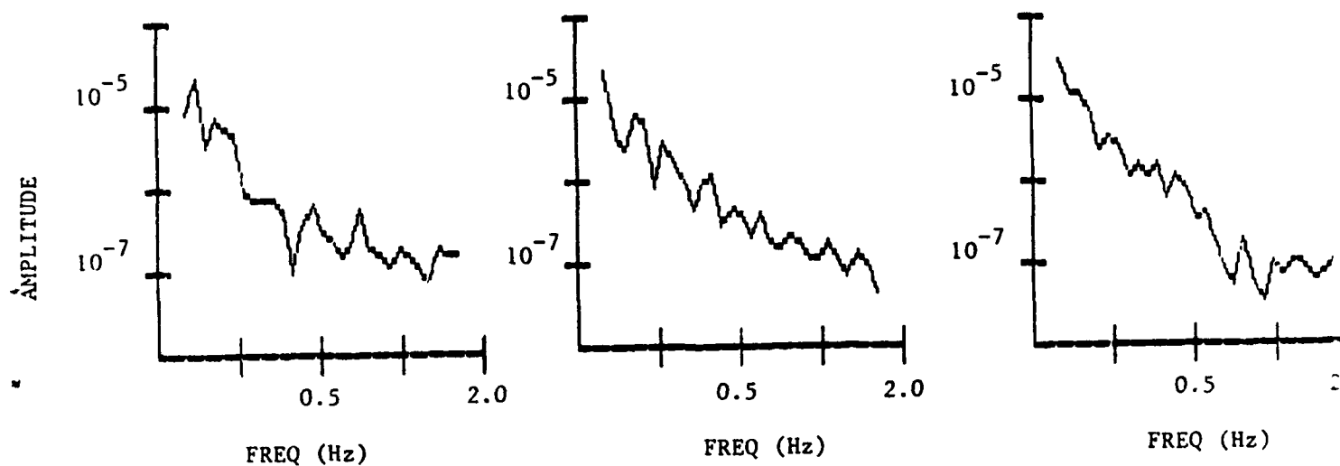
Li wave
