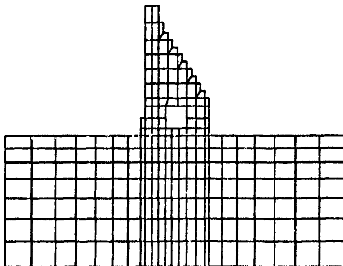
b. Finite element mesh
