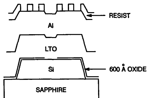
(d) Photo step for contacts.
