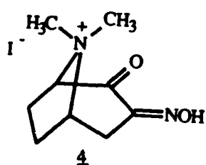
(+)-3-Oximino-tropan-2-one methiodide
