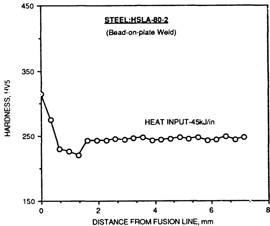
Fig. B-11. HAZ hardness profile. Steel : HSLA-80-2. Heat Input : 45 kJ/in
