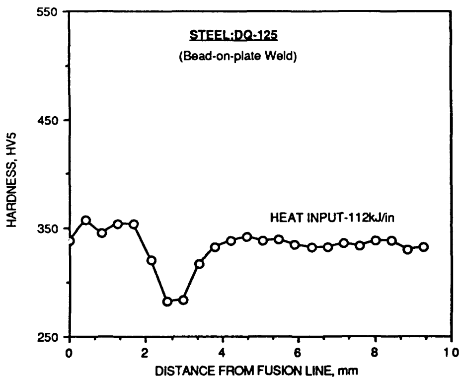
Fig. B-30. HAZ hardness profile. Steel : DQ-125. Heat Input : 112 kJ/in
