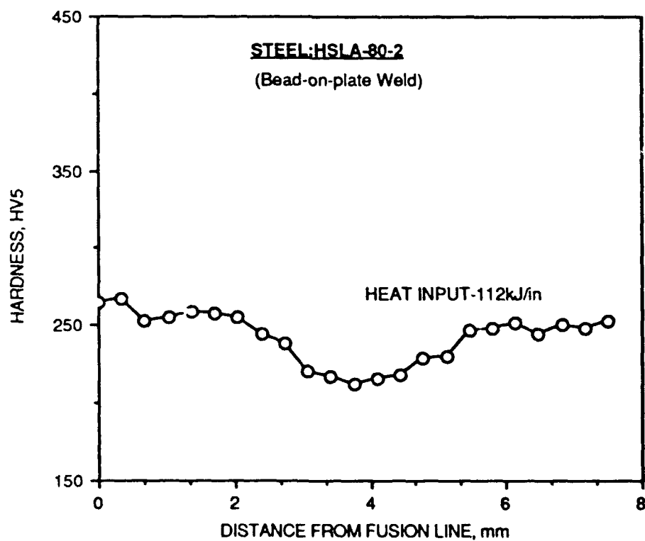
Fig. B-14. HAZ hardness profile. Steel : HSLA-80-2. Heat Input : 112 kJ/in
