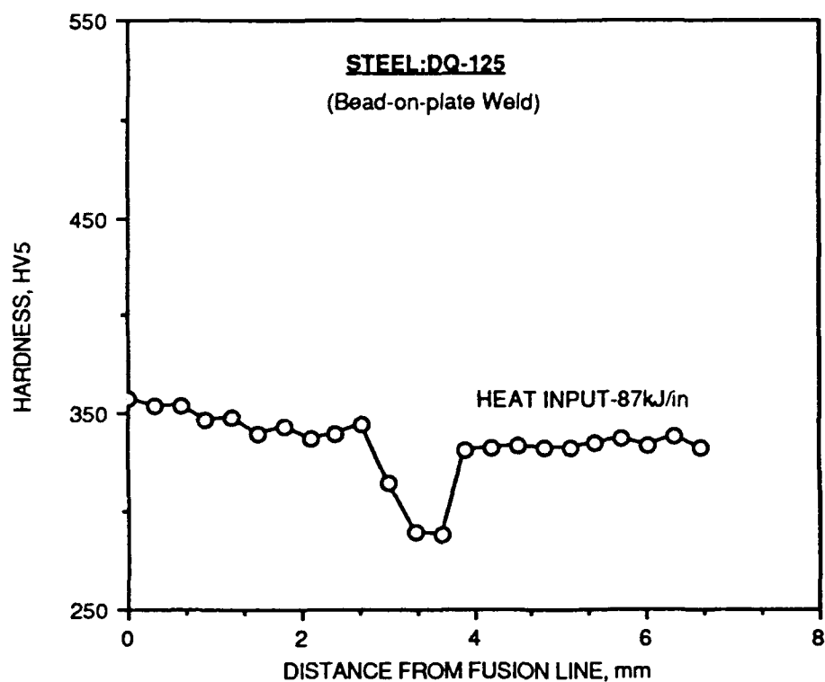
Fig. B-29. HAZ hardness profile. Steel : DQ-125 Heat Input : 87 kJ/in
