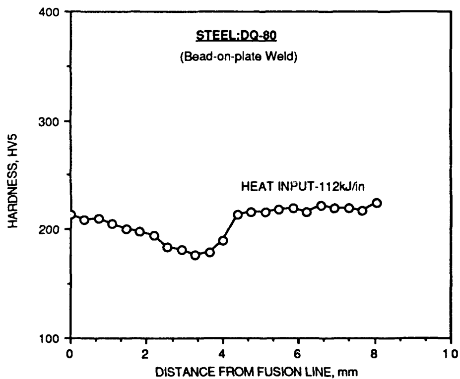
Fig. B-22. HAZ hardness profile. Steel : DQ-80. Heat Input : 112 kJ/in
