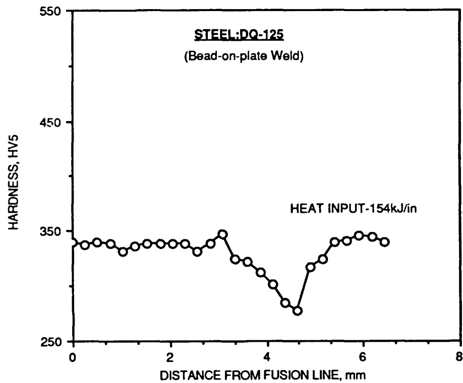
Fig. B-31. HAZ hardness profile. Steel : DQ-125. Heat Input : 154 kJ/in
