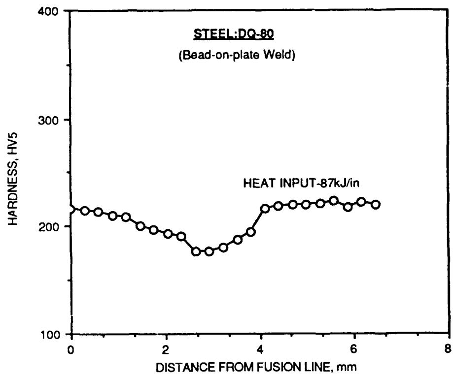
Fig. B-21. HAZ hardness profile. Steel : DQ-80. Heat Input : 87 kJ/in
