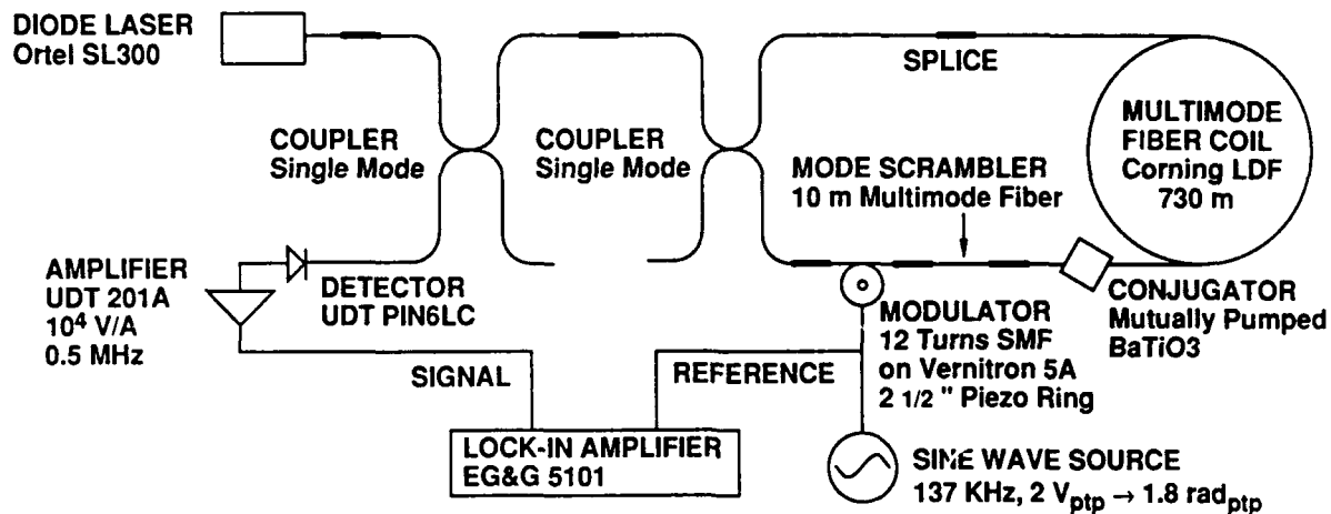
Fig. 3 All-fiber PCFOG.
