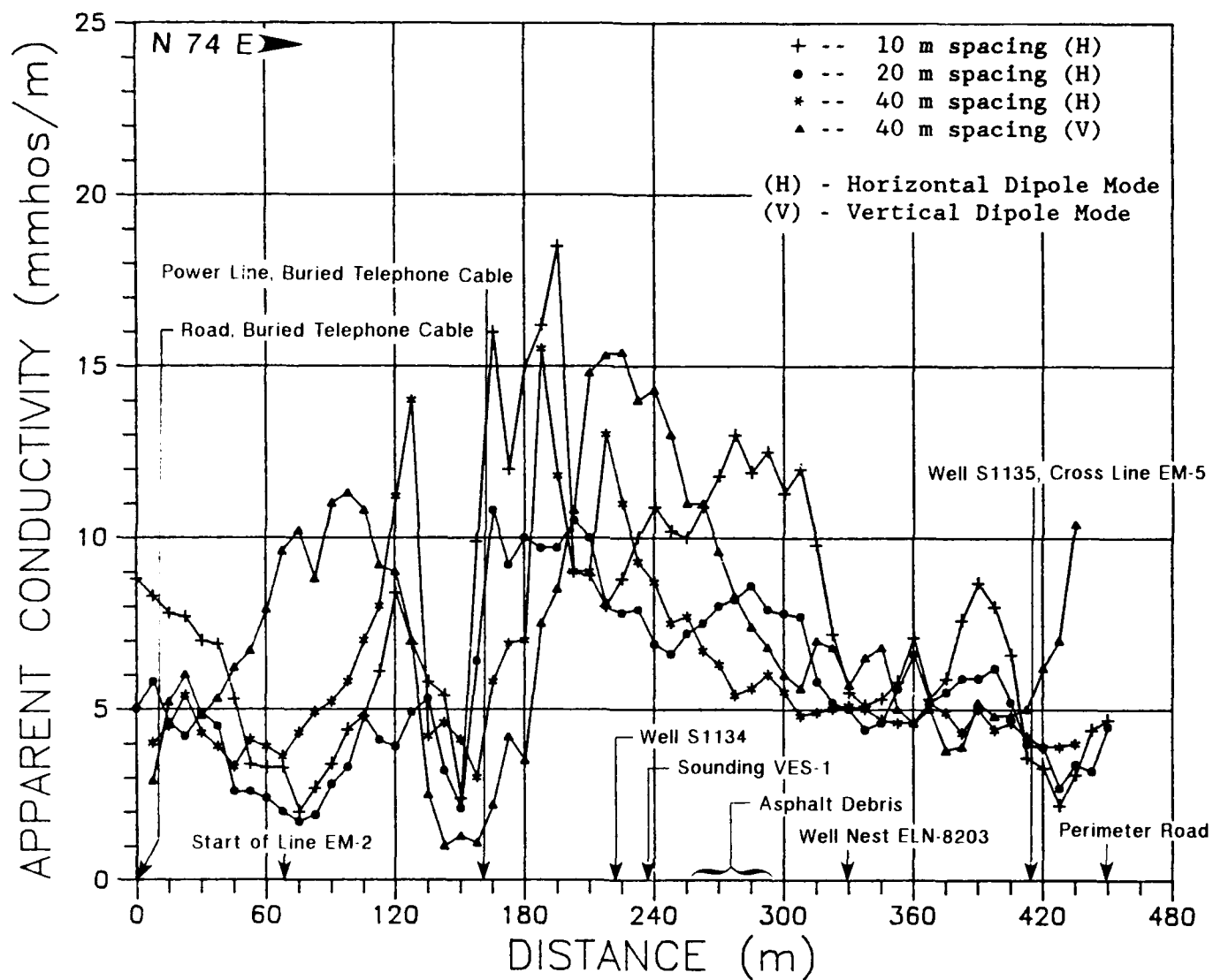
Figure 9. Results of EM survey line EM-1
