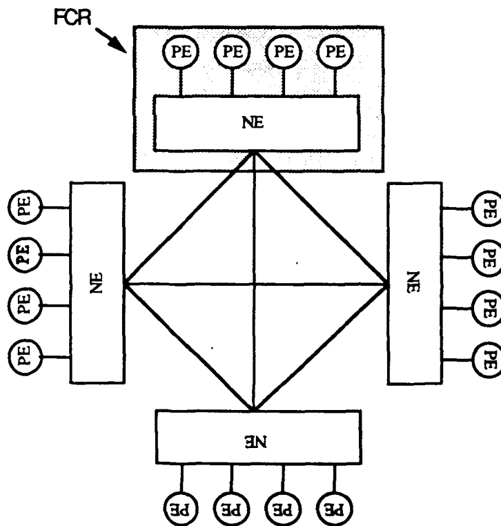
Figure 2-3. The FTTP
