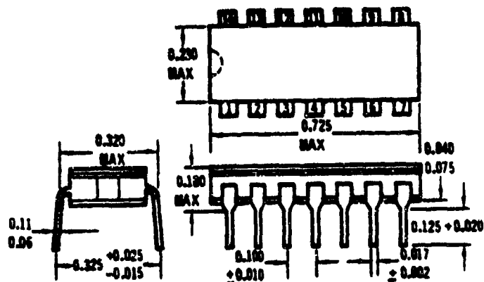
14 Lead Cavity DIP (D)
