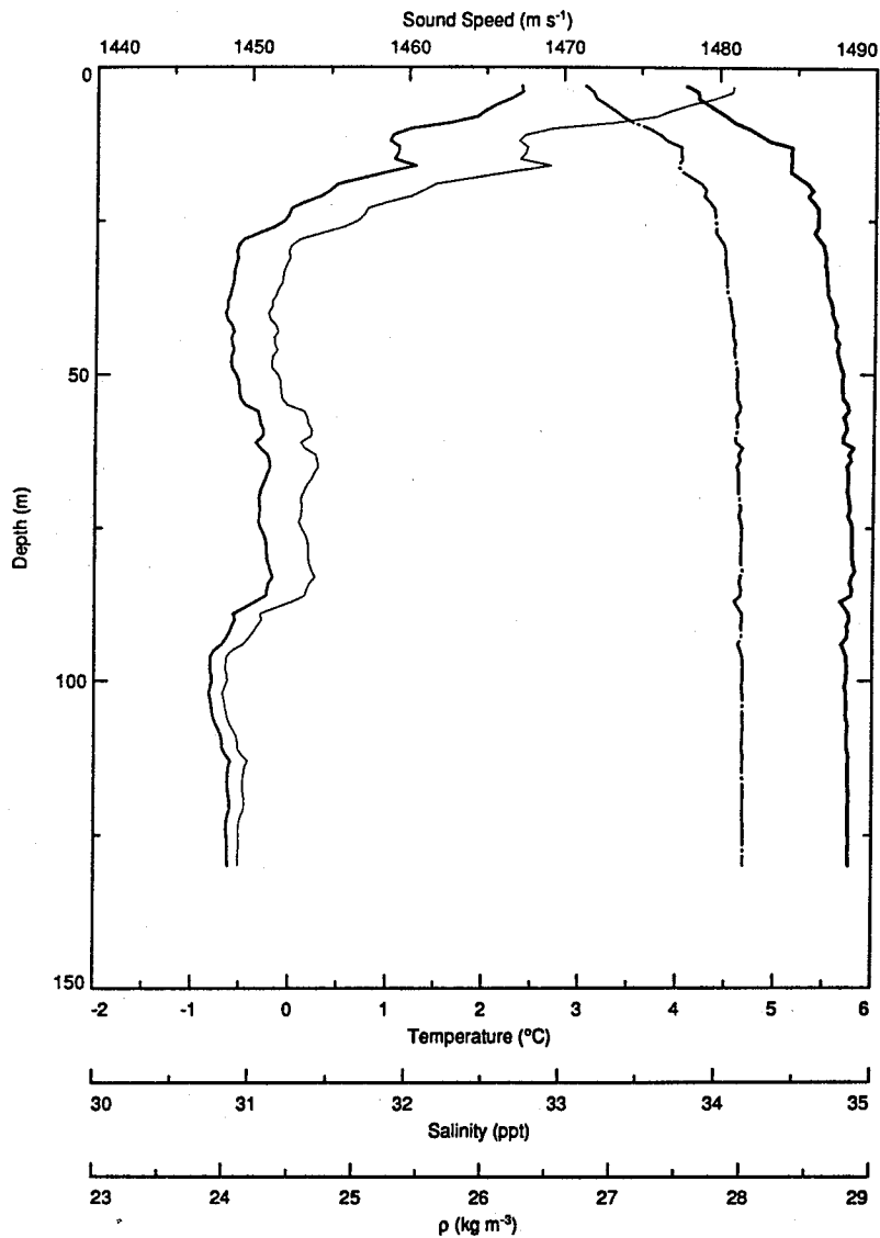
1989 MST : CTD Cast 031
