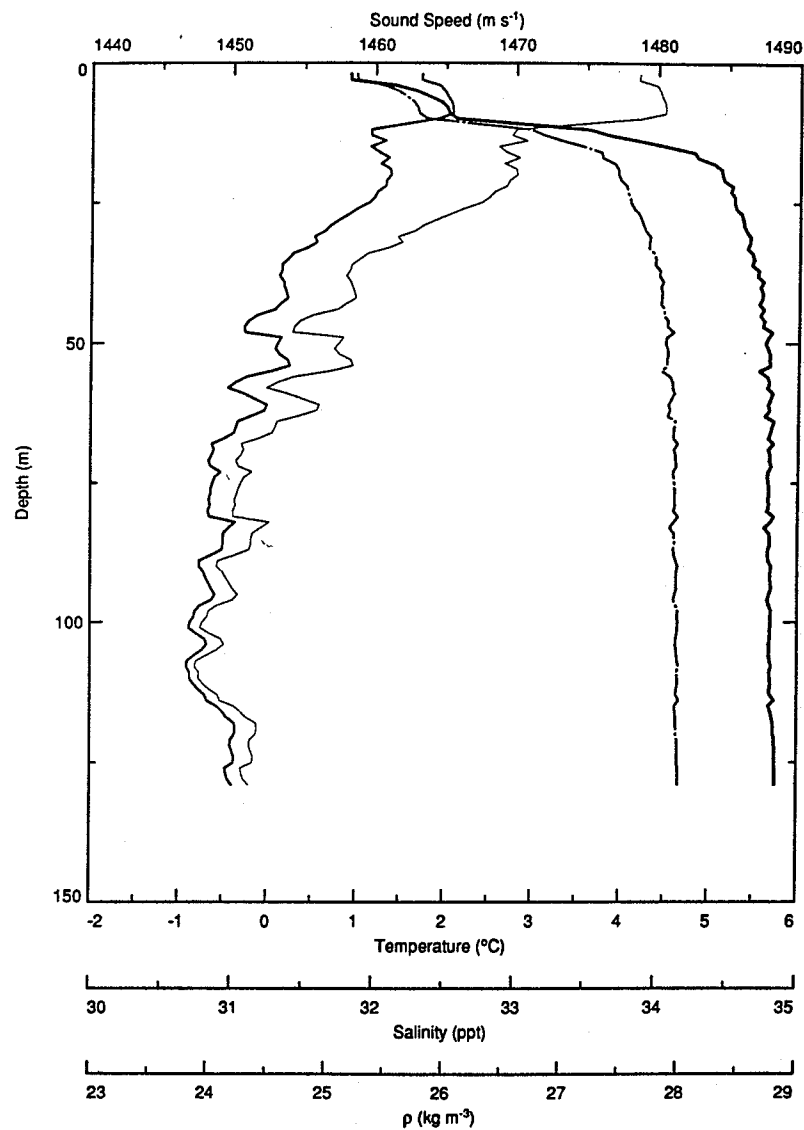
1989 MST : CTD Cast 052
