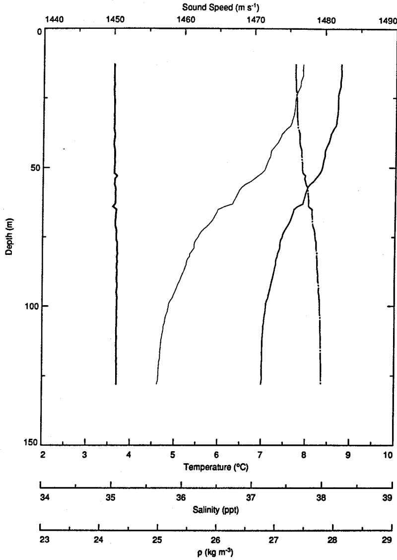
1989 MST : CTD Cast 001
