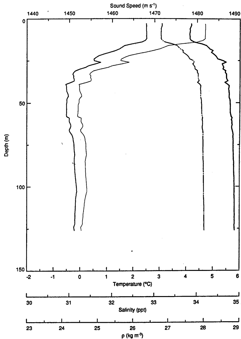
1989 MST : CTD Cast 045
