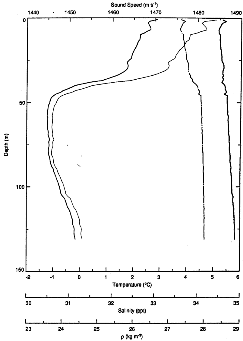
1989 MST : CTD Cast 038
