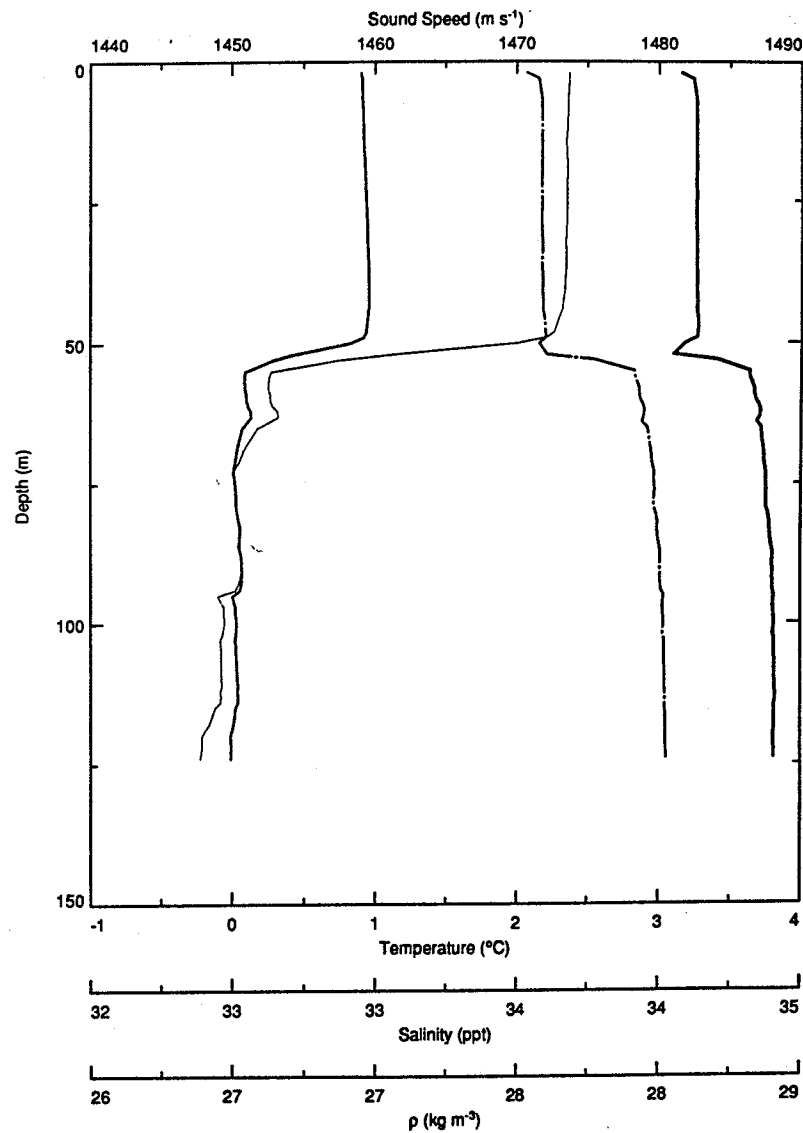
1988 MST : CTD Cast 014
