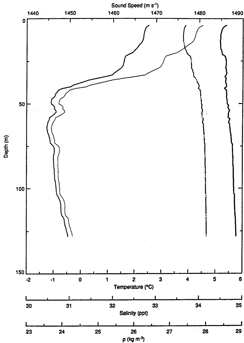
1989 MST : CTD Cast 037
