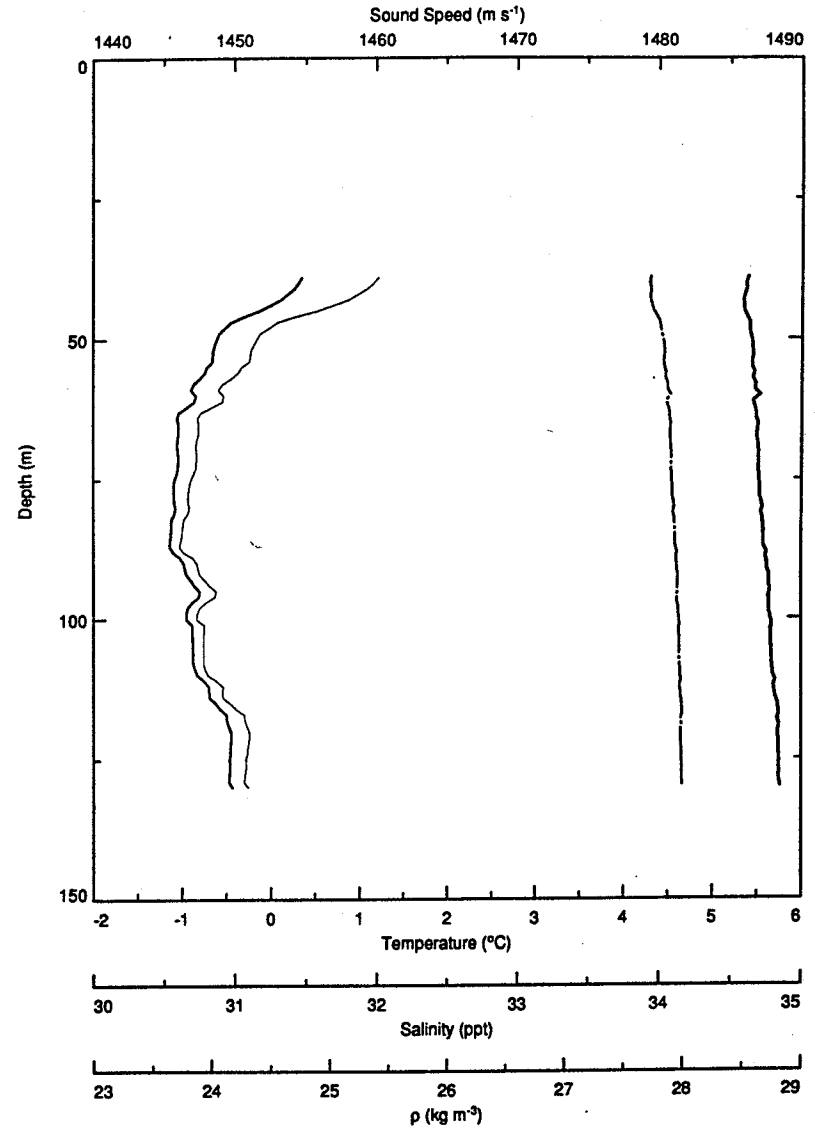
1989 MST : CTD Cast 017
