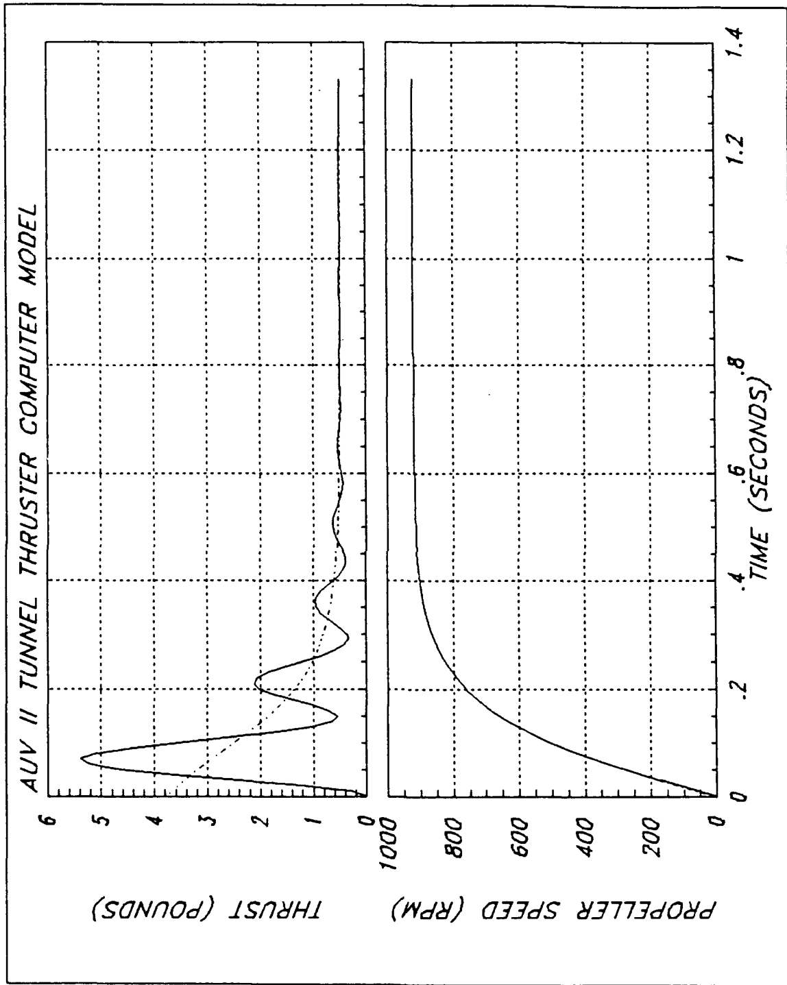
Figure 15 24 Volt Baseline
