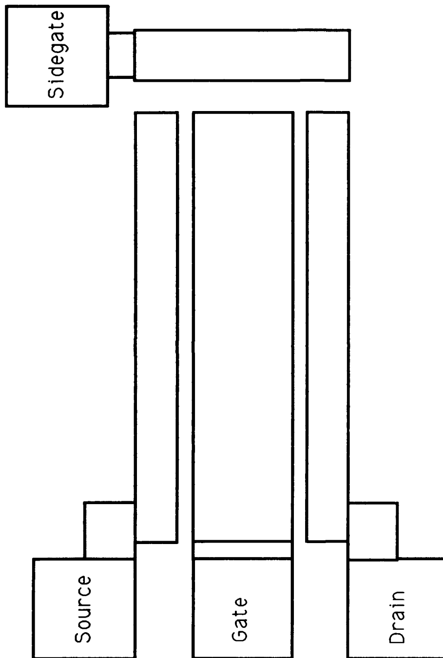
Fig. 2-4. 100 x 400um FET Layout
