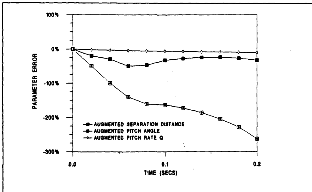
Figure 20 Parameter Error (Augmented)
