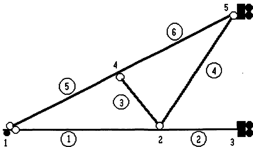
Fig. 3.4 TRUSS 4
