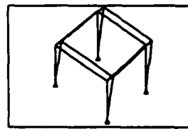
Mode 2 (136 Hz)
