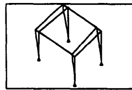
Mode 1 (131 Hz)
