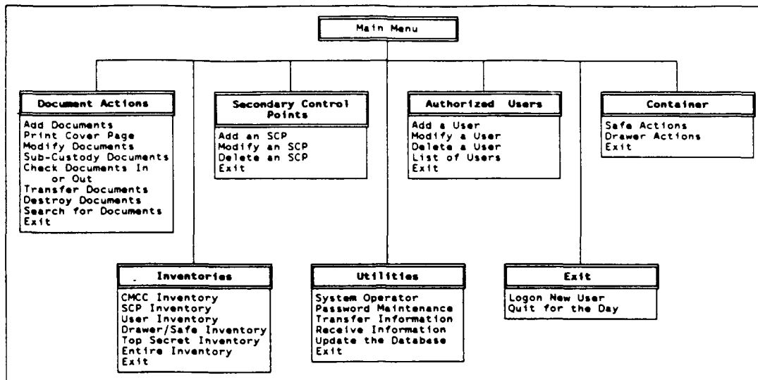
Figure 9a. Main Menu Hierarchy.
