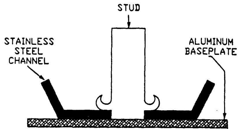
'FRICTION' RIVET
