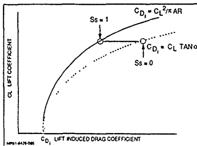
Fig. 56 S_s Parameter Definition
