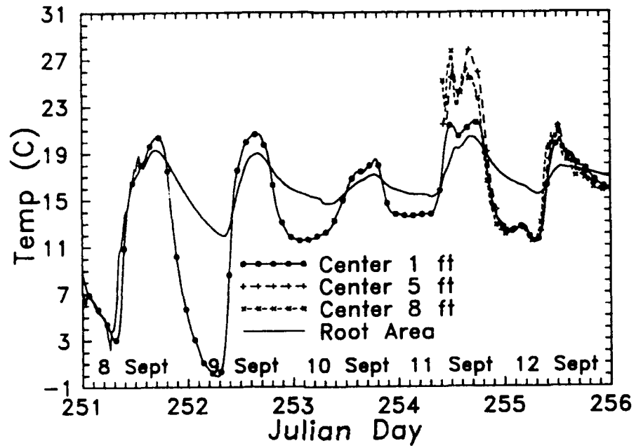
Figure B-1. (Cont.) (g.) Center Temperatures
