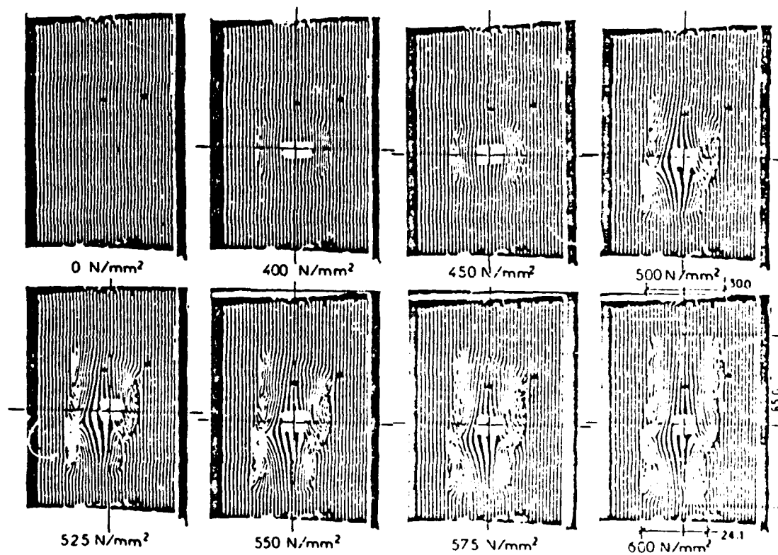
Fig: 2- VISUALISATION DU DELAMINAGE (DLR)
