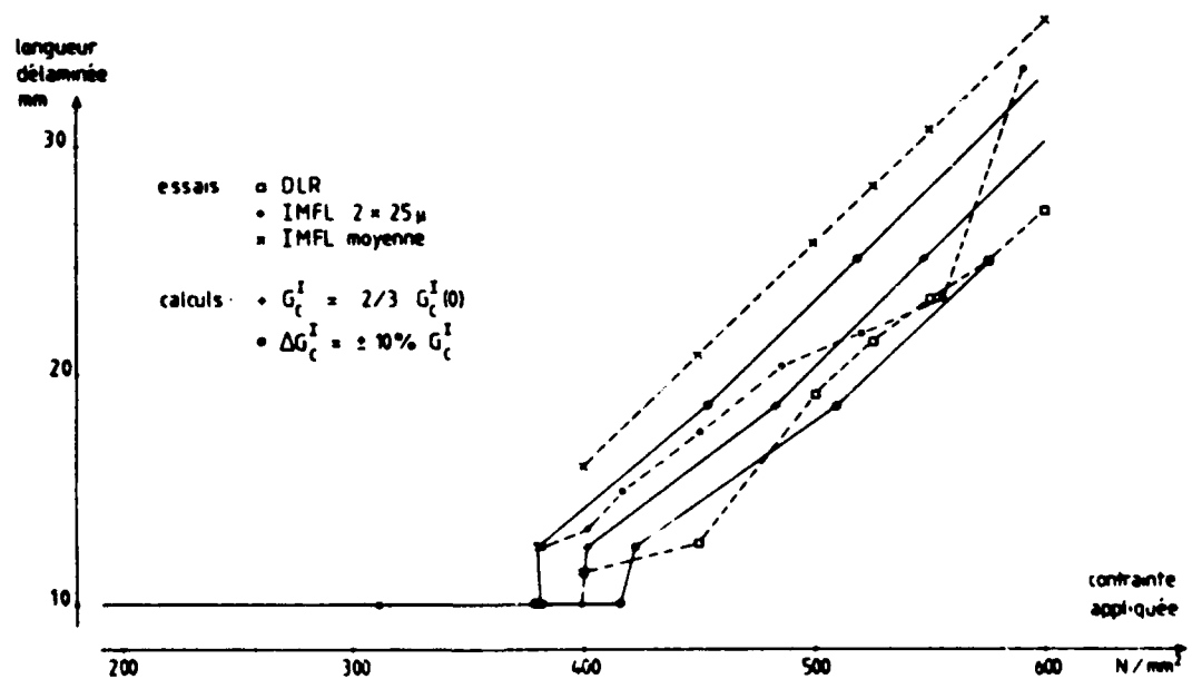
Fig 6 - Propagation du délaminage (komparason essais-calculs)
