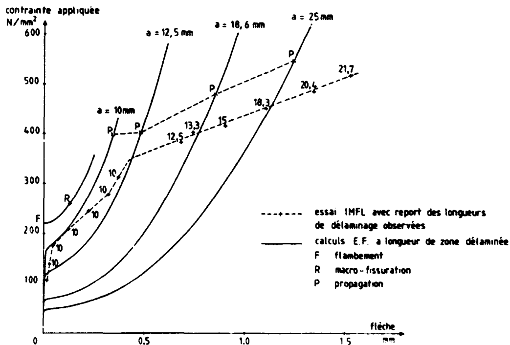
Fig. 4 - Flèche au centre de la zone délaminée
