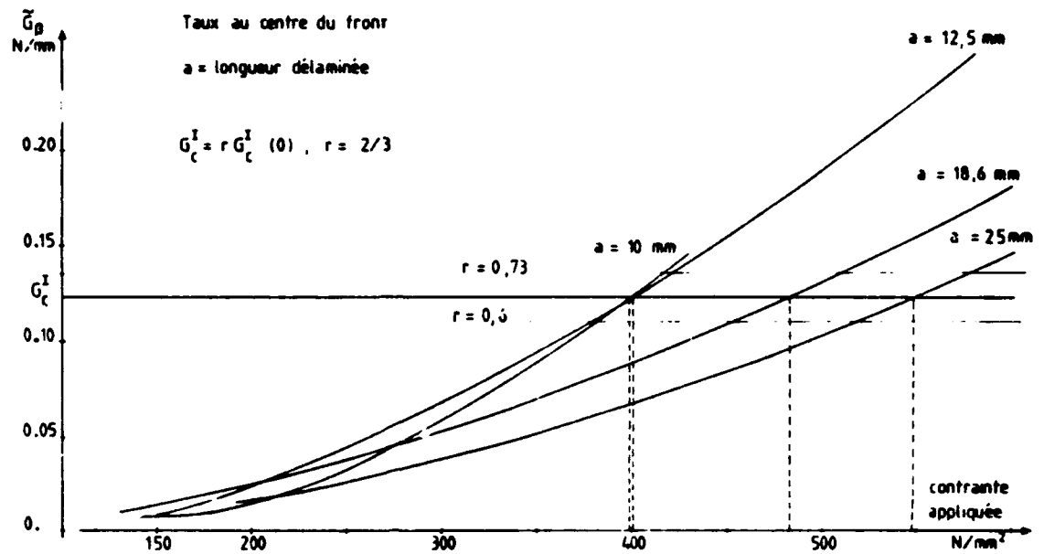
Fig 5 - Evolution du taux de restitution d'énergie
