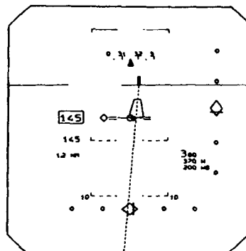
Figure 13 : Collimateur tête haute du CEV.
